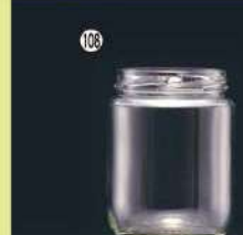
108 ジャム300ST瓶 70φ×H93(252ml) 72入 口部:63ツイスト 材質ガラス
