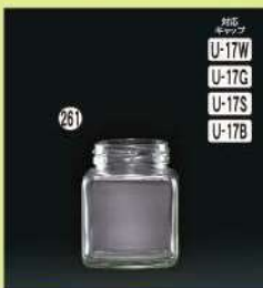
261 50角ツイスト 49.5φ×H64(93ml) 108入 口部:43ツイスト 材質ガラス
