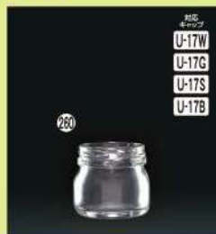
260 SIジャム35 45φ×H40.2(35ml) 240入 口部:43ツイスト 材質ガラス
